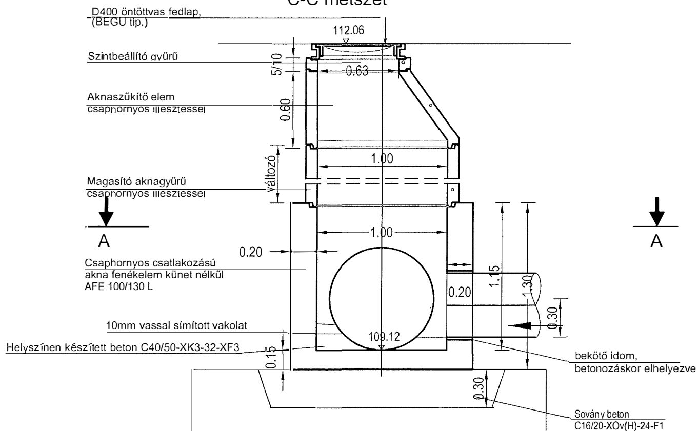
C-C metszet
